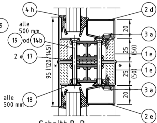
Schnitt B-B
