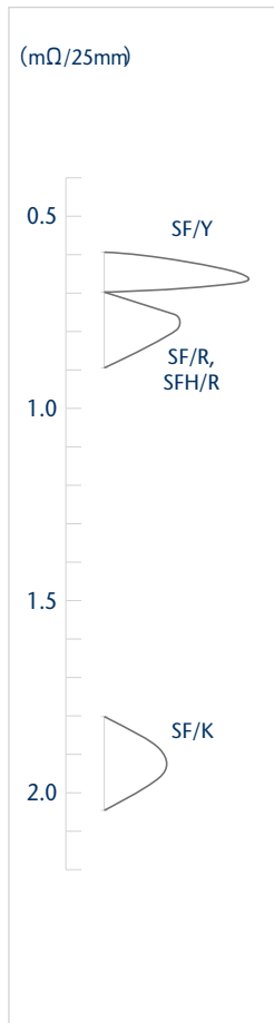
Resistencia interna
