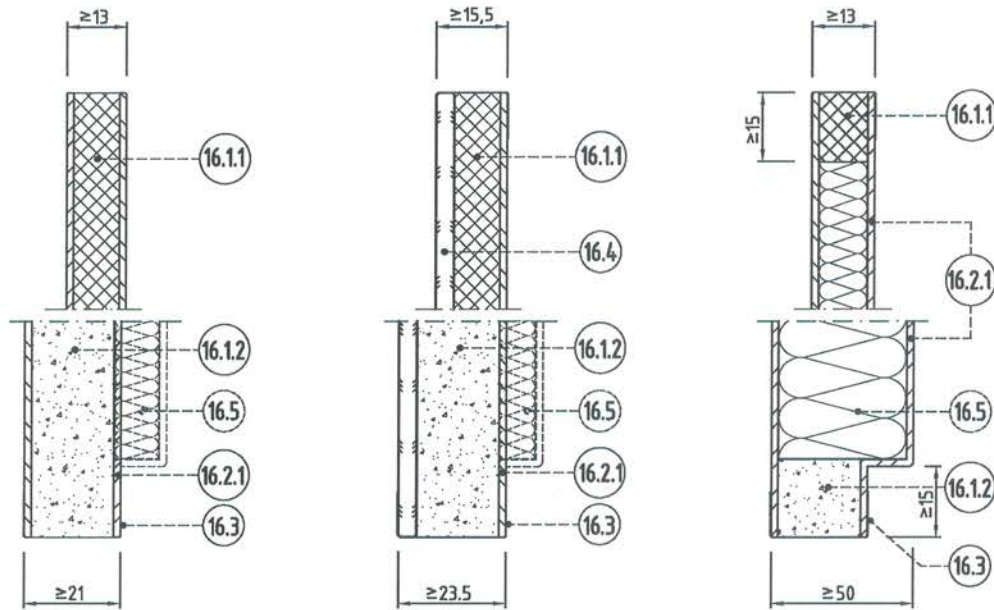
Abmessungen der Ausfüllungen bis max. 1250 mm x 2000 mm
