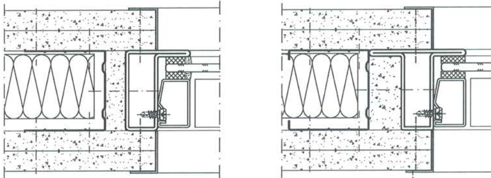
Deckschalen wahlweise aus Stahl, Aluminium oder Holz \geq 1,0 mm dick
